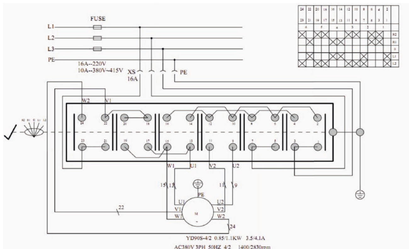
Schéma électrique
