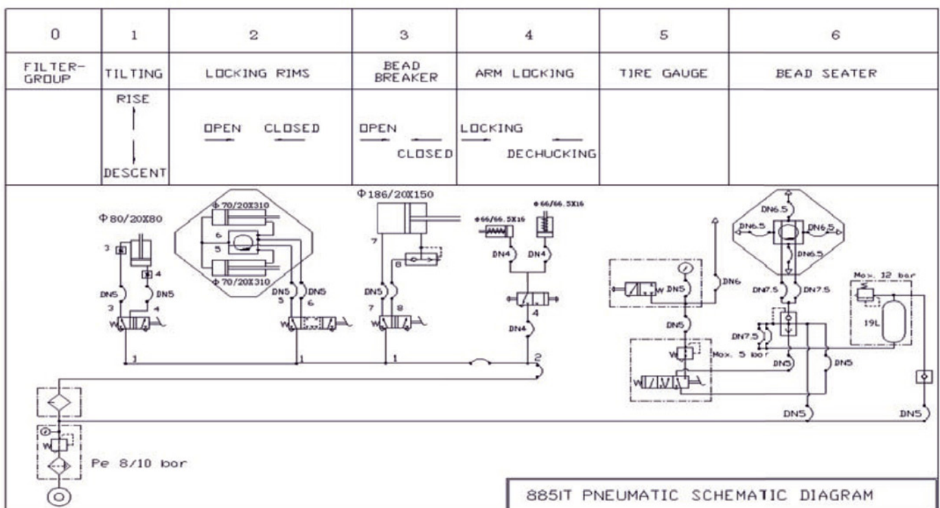
Pneumatiskt diagram
