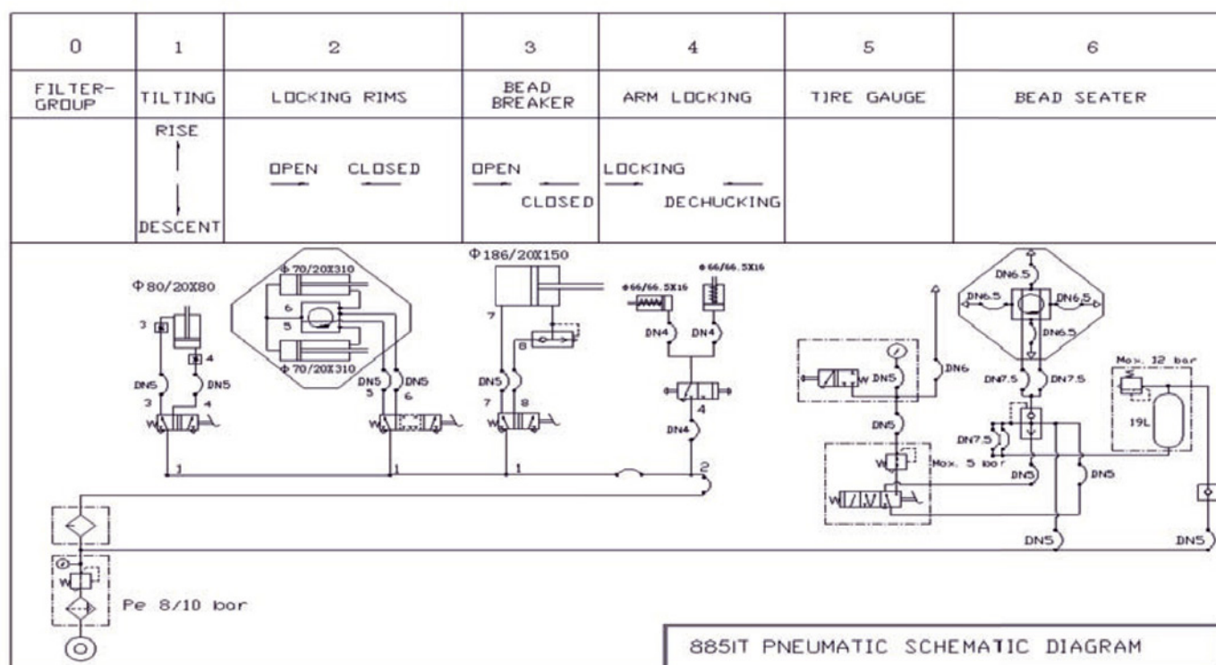
Schéma pneumatique
