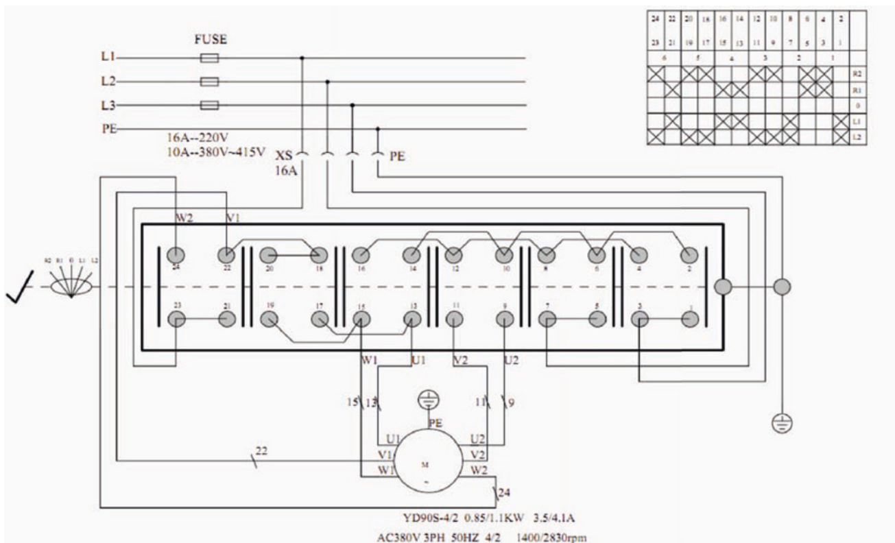
Elektriskt diagram
